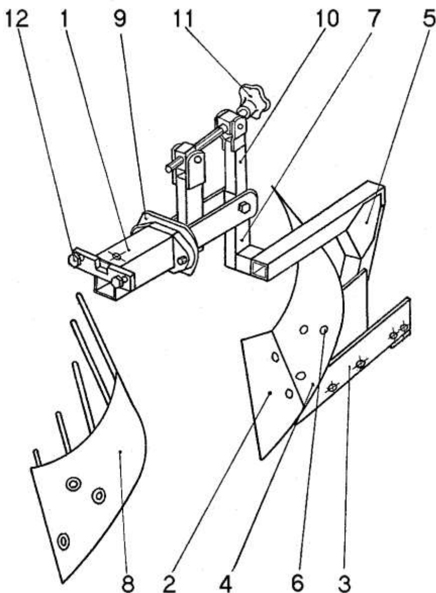
Рисунок 1 – Плуг ПУ-00.000-01
