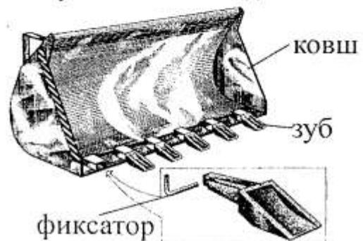
Рисунок 1.11 – Ковш
