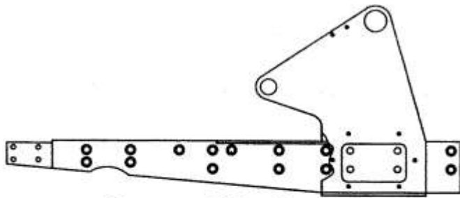
Рисунок 2.1 – Рама
