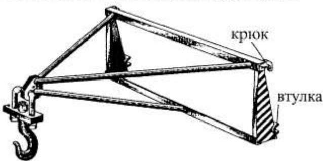
Рисунок 1.6 – Крюк монтажный
