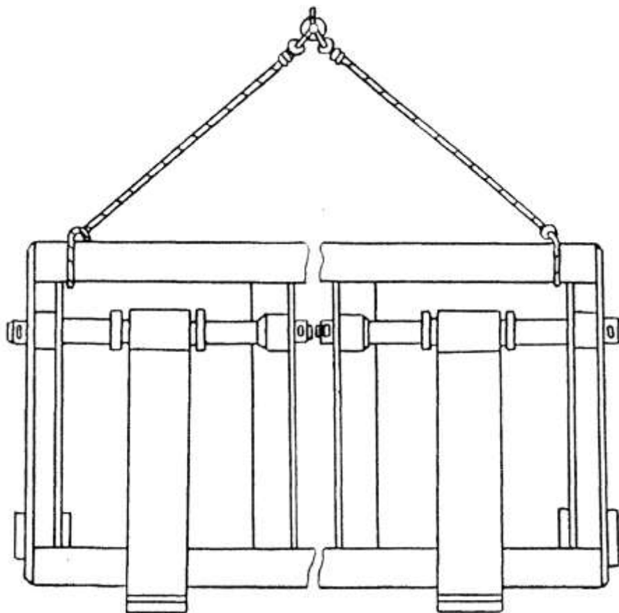
Рисунок 7.6 – Схема строповки вил грузовых
