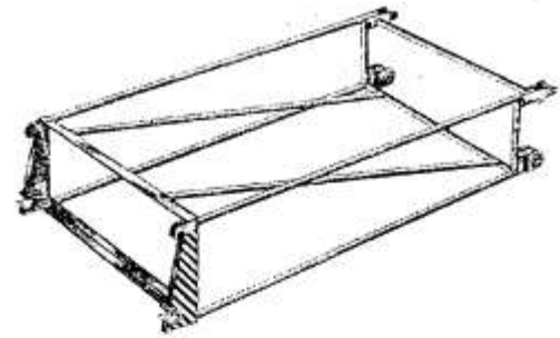
Рисунок 1.3 – Удлинитель
