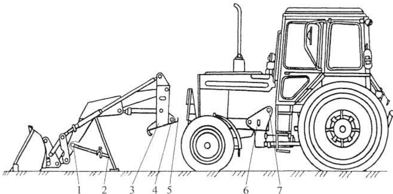
Рисунок 3.2 – Оборудование рабочее съемное 1 – труба стрелы; 2 – опора; 3 – портал; 4 – зажим; 5 – болт; 6 – рама; 7 — палец
