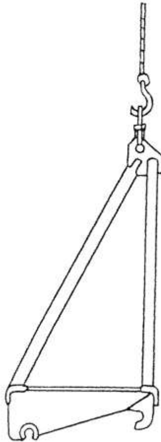
Рисунок 7.4 – Схема строповки крюка монтажного
