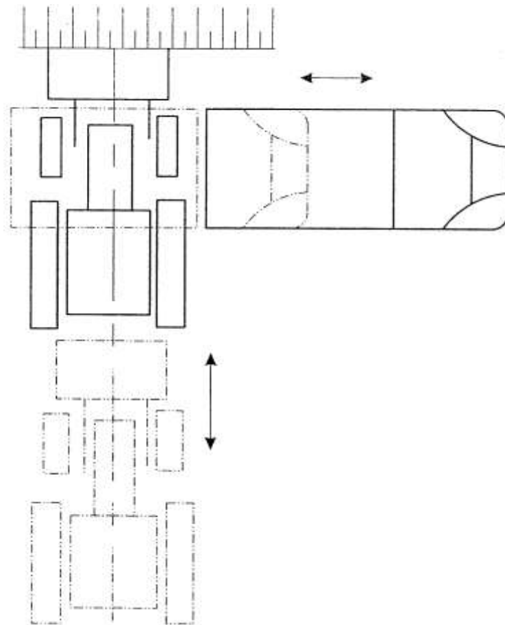
Рисунок 3.4 – Схема челночного способа работы
