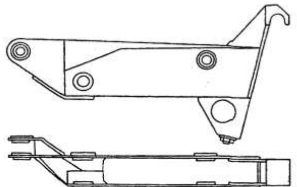
Рисунок 2.6 – Портал
