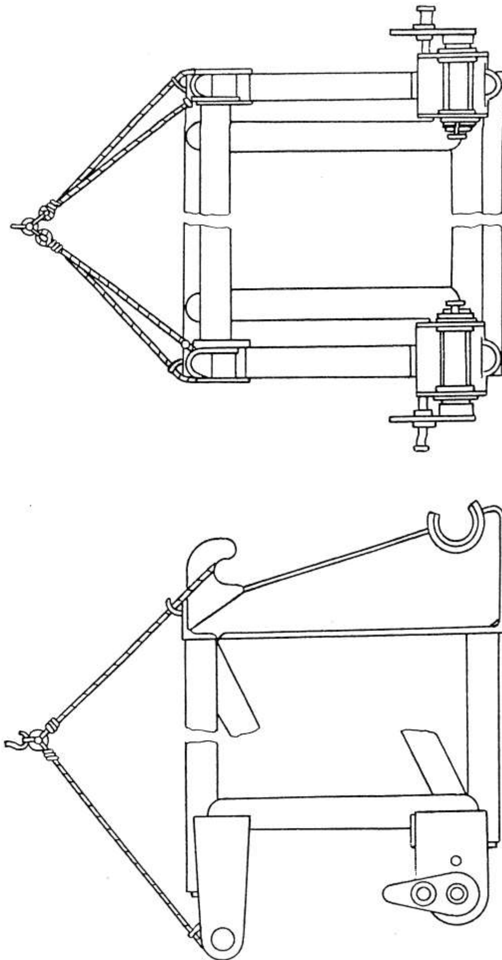
Рисунок 7.7 – Схема строповки удлинителя
