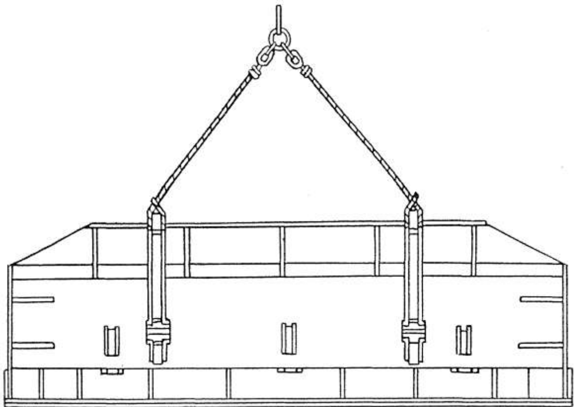
Рисунок 7.2 – Схема строповки отвала
