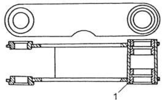
Рисунок 2.9 – Рычаг
