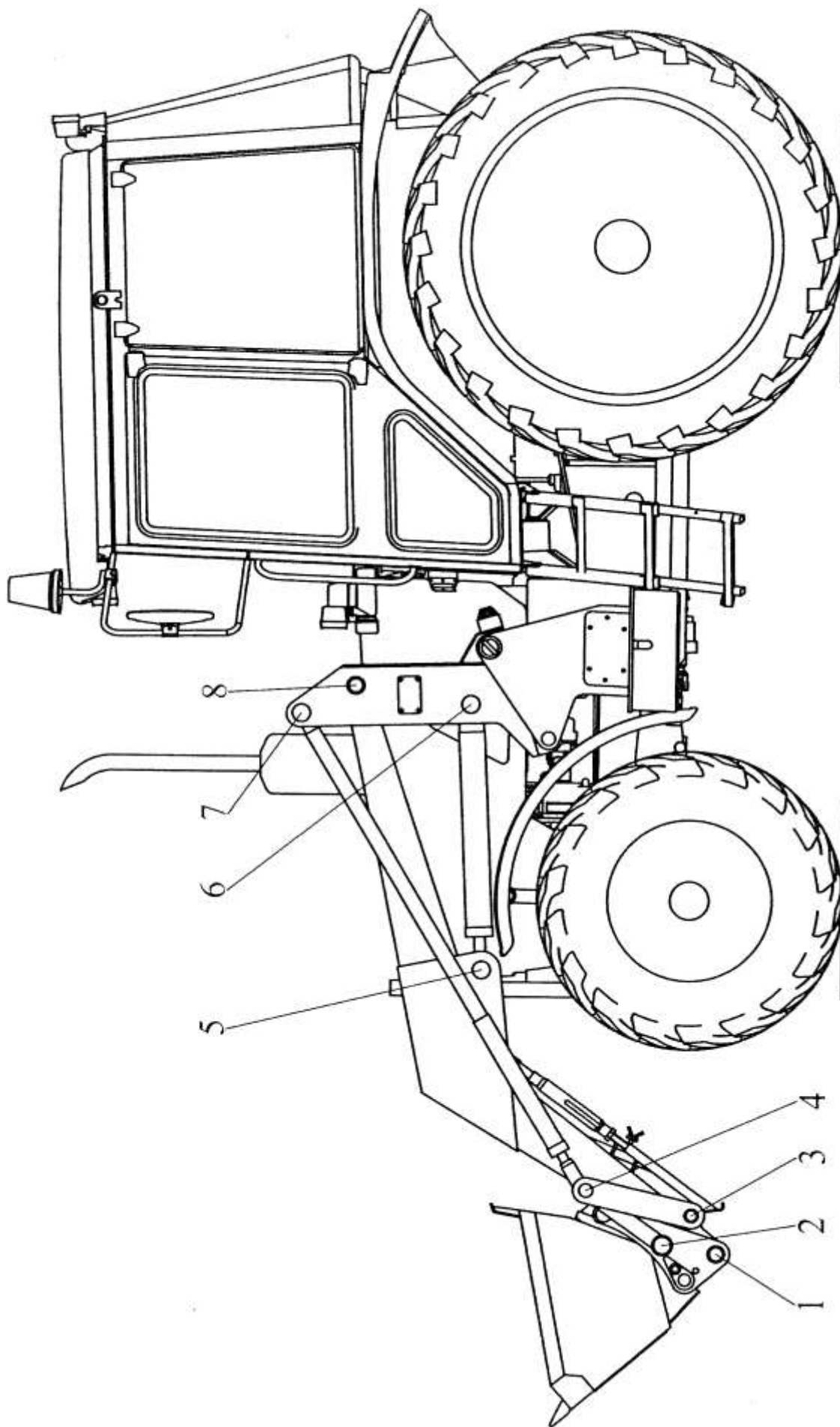
Рисунок 4.1 – Схема смазки оборудования
