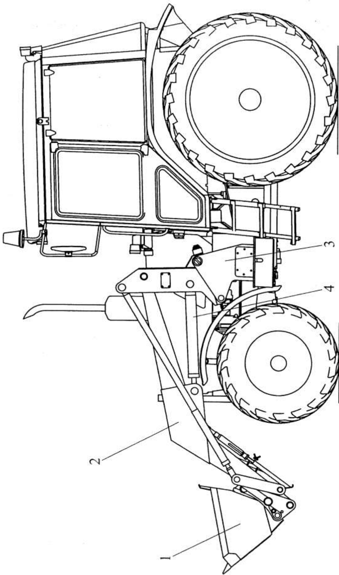
Рисунок 1.1 – Оборудование рабочее погрузчика П10М
