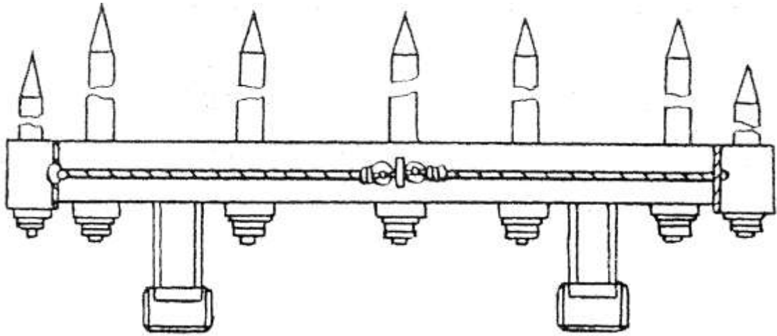
Рисунок 7.3 – Схема строповки вил сельскохозяйственных
