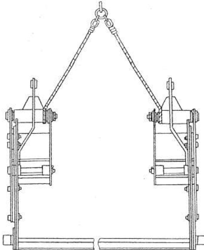
Рисунок 7.5 – Схема строповки ковша двухчелюстного
