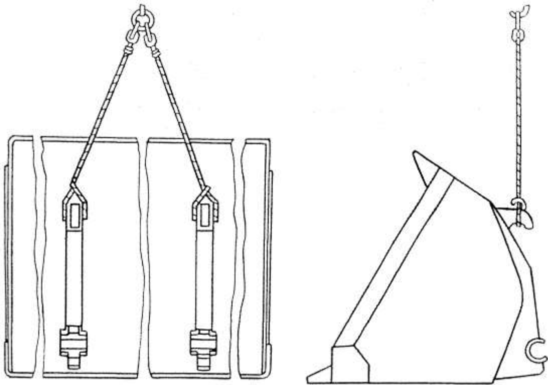
Рисунок 7.1 – Схема строповки ковша, ковша увеличенного, ковша для снега, ковша для корнеплодов
