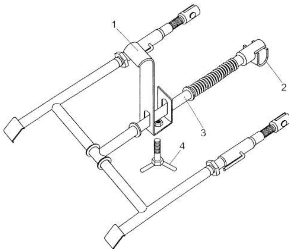
Рисунок 3.1 – Опора
