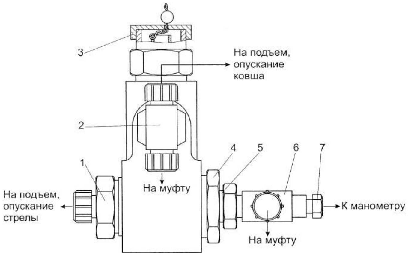
Рисунок 2.11 – Клапан предохранительный 1 – штуцер; 2 – тройник ввертной; 3 – крышка; 4 – переходник ввертной; 5 – шайба защитная; 6 – тройник; 7 – пробка
