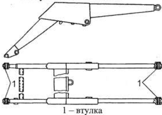
Рисунок 2.5 – Стрела
