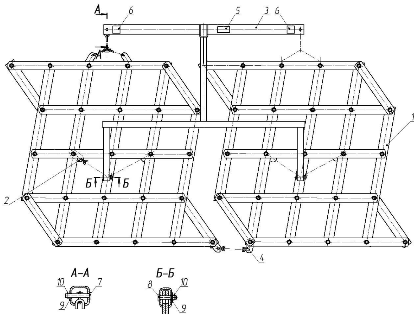
Рисунок 1 – Борона тракторная БТ-1.6
