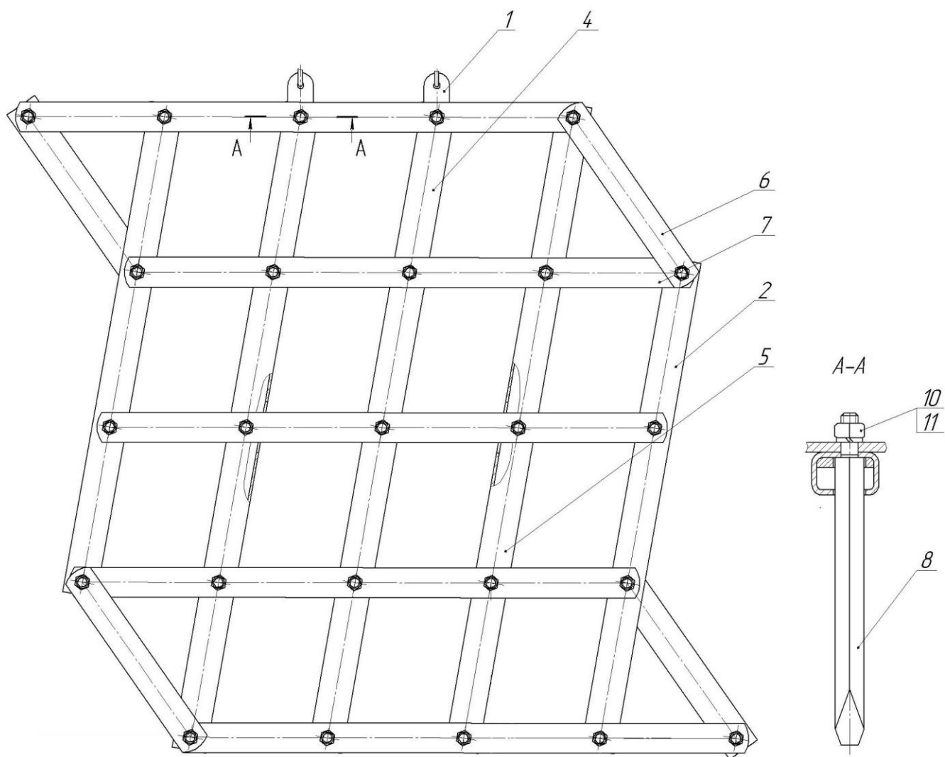
Рисунок 2 – Борона
